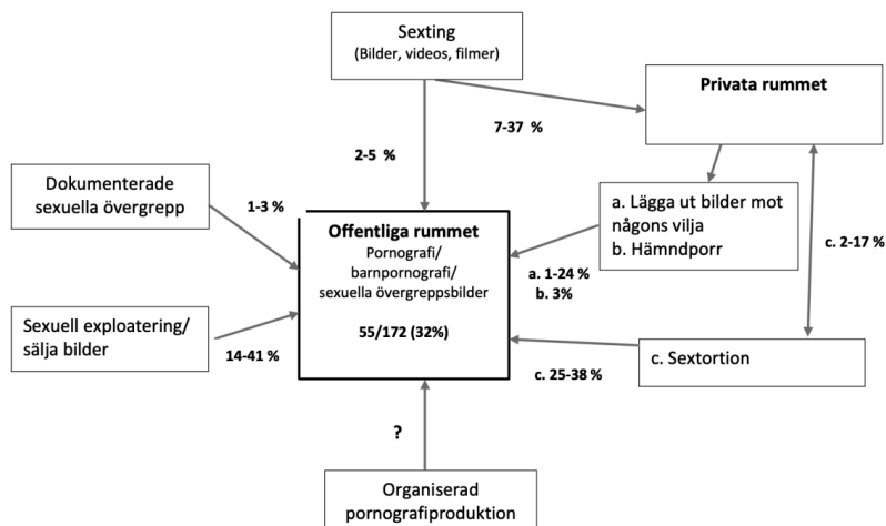
Figur 3. Resultatmodell
